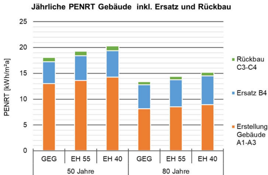
Abbildung 16: Jährliche PENRT inkl. Ersatz und Rückbau für das Gebäude
