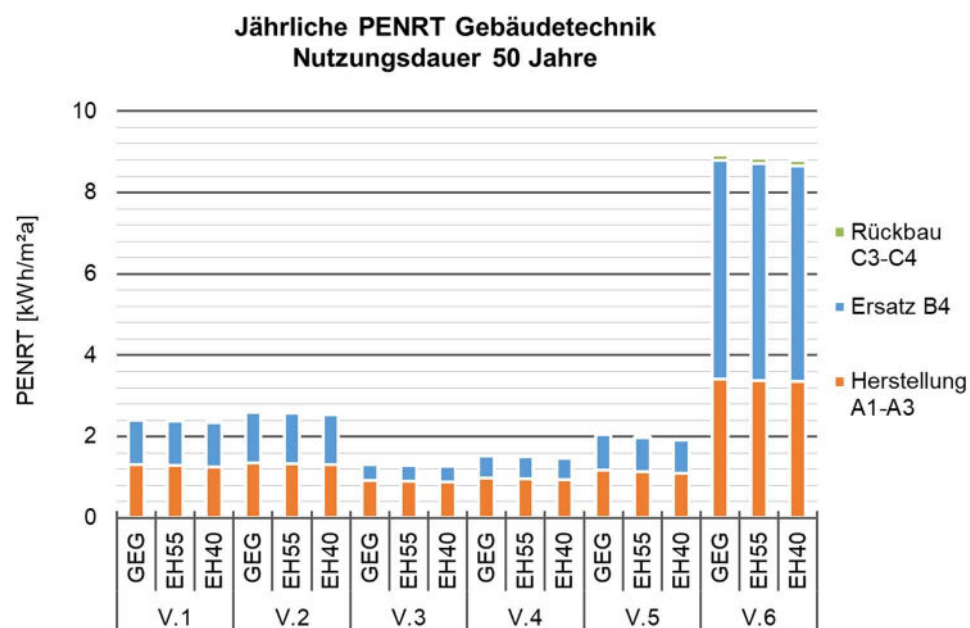
Abbildung 18: Jährliche PENRT Gebäudetechnik für Nutzungsdauer 50 Jahre
