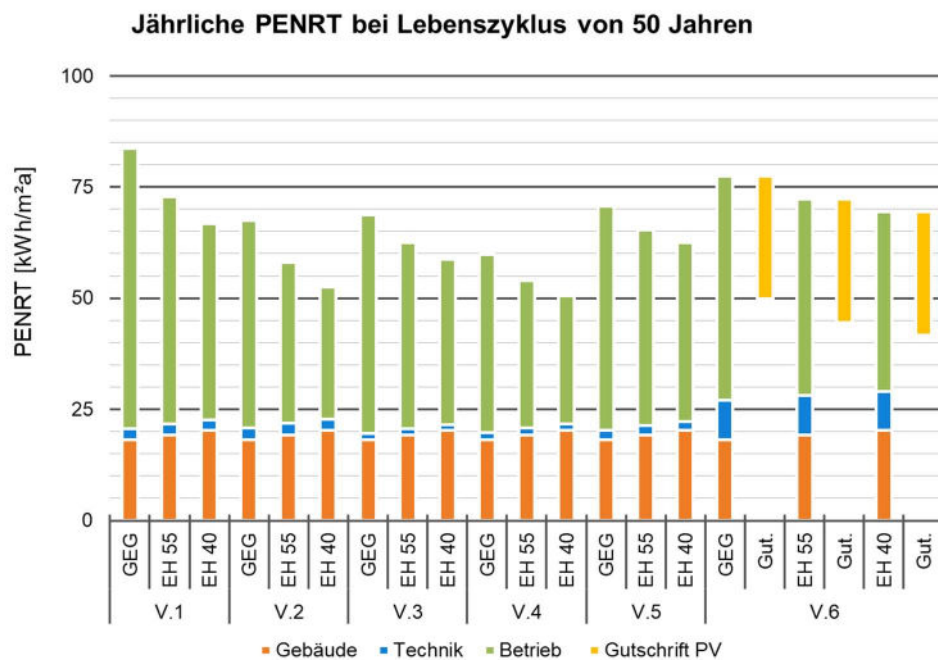
Abbildung 24: Jährliche PENRT über gesamten Lebenszyklus
