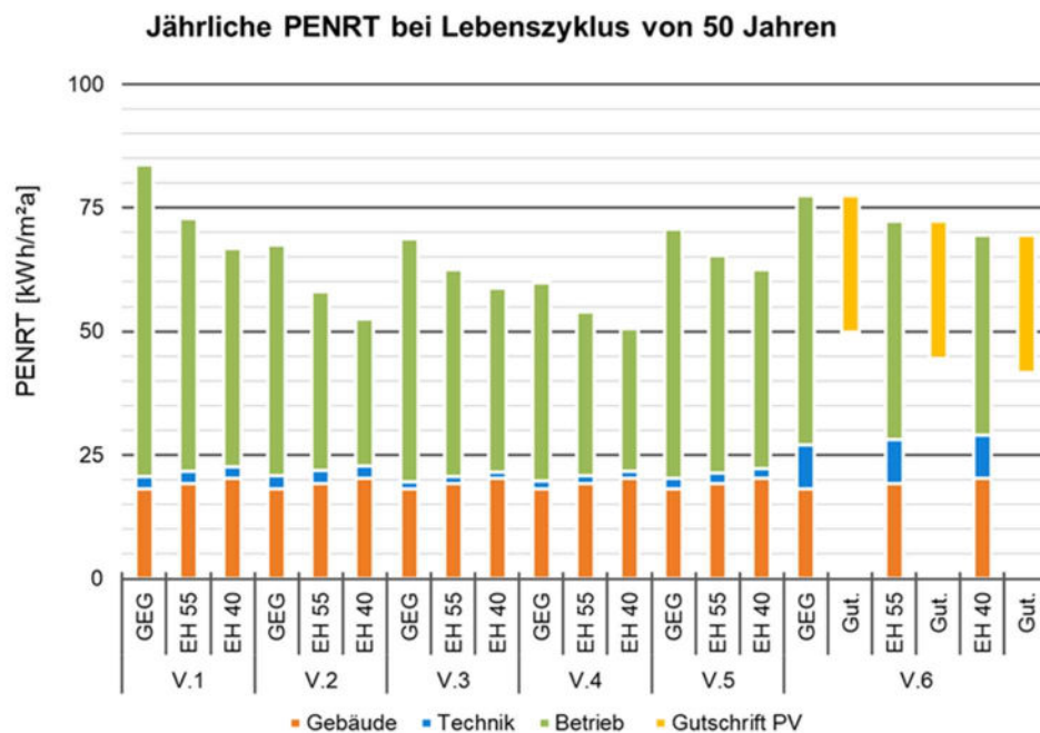
Abbildung 2: PENRT über den gesamten Lebenszyklus pro m² Nutzfläche für 50 Jahre Nutzungsdauer
