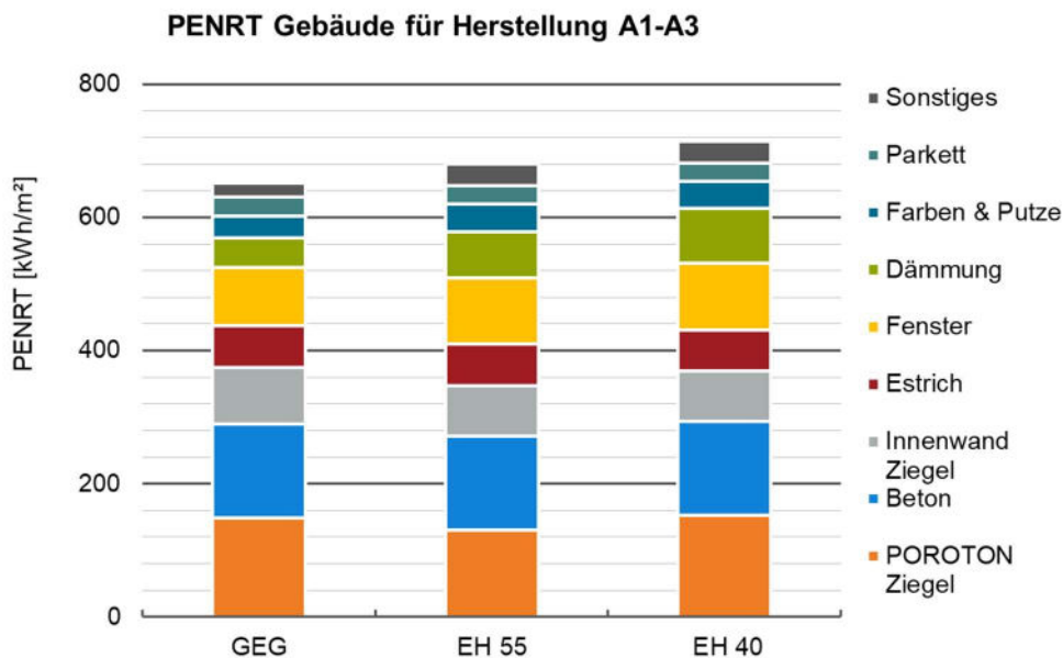
Abbildung 14: PENRT Herstellungsphase A1-A3 für das Gebäude nach Material
