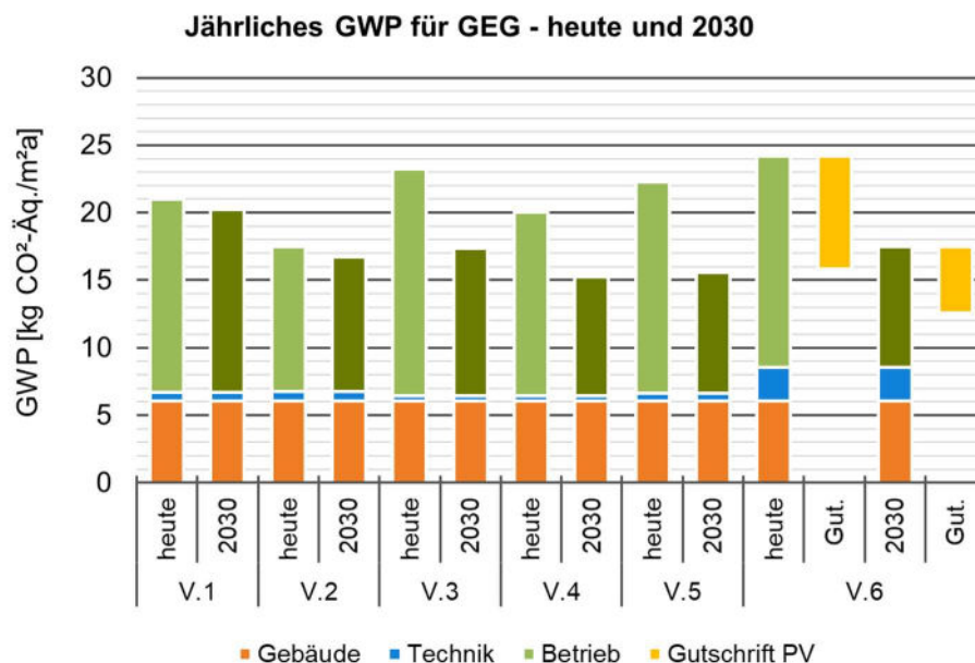
Abbildung 29: Jährliches GWP für GEG - Zukunftsszenario
