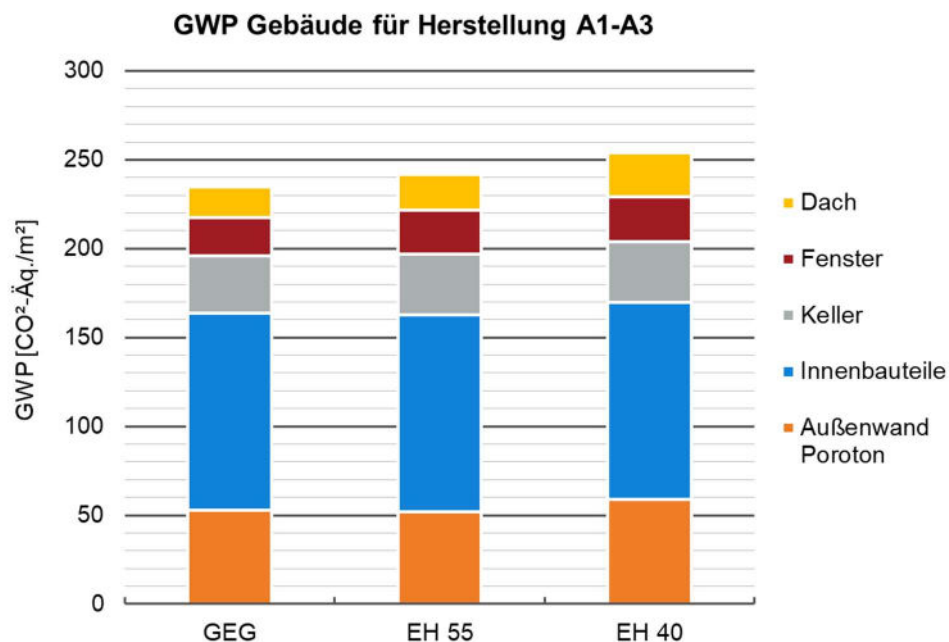
Abbildung 11: GWP Herstellungsphase A1-A3 für das Gebäude nach Bauteilen
