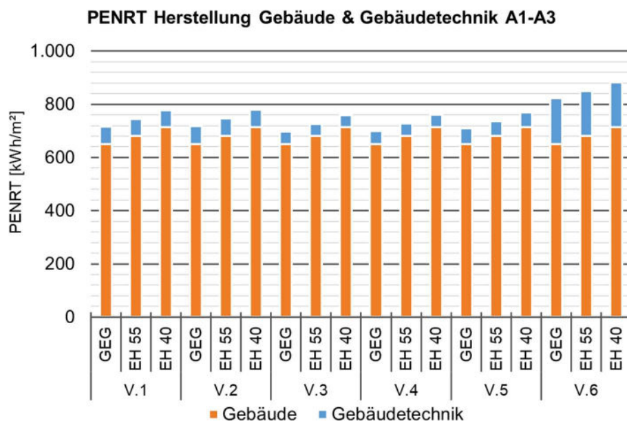
Abbildung 20: PENRT Herstellungsphase A1-A3 für Gebäude & Gebäudetechnik
