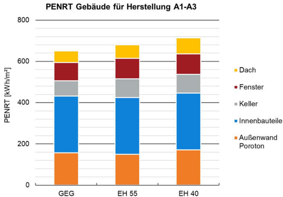
Abbildung 12: PENRT Herstellungsphase A1-A3 für das Gebäude nach Bauteilen
