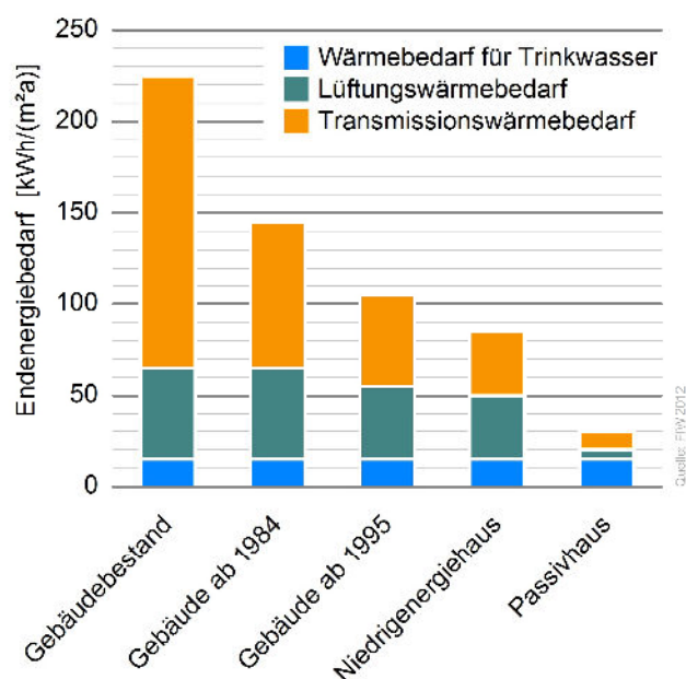
Abbildung 4: Entwicklung des Energiesparenden Bauens in Deutschland und Anteile an den Wärmeverlusten – mittlerer Endenergiebedarf typischer EFH-Wohngebäude
