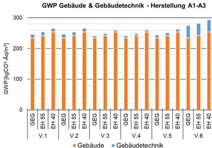
Abbildung 19: GWP Herstellungsphase A1-A3 für Gebäude und Gebäudetechnik
