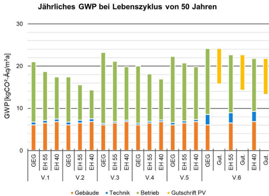
Abbildung 23: Jährliches GWP über gesamten Lebenszyklus
