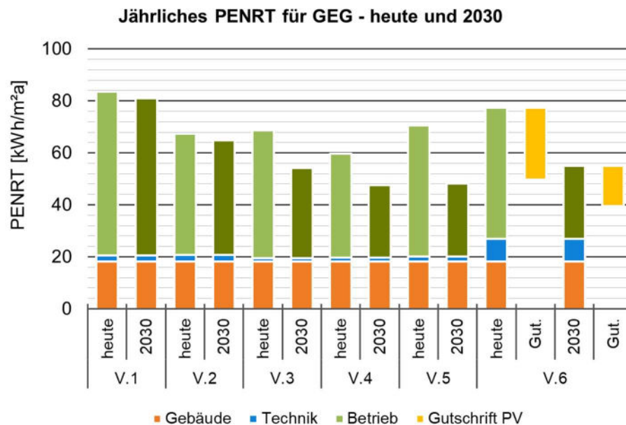
Abbildung 30: Jährliche PENRT für GEG - Zukunftsszenario
