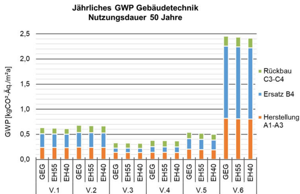
Abbildung 17: Jährliches GWP Gebäudetechnik für Nutzungsdauer 50 Jahre
