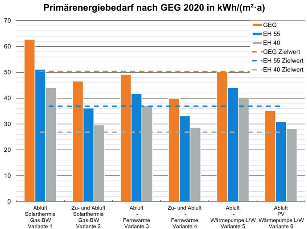
Abbildung 10: Primärenergiebedarf der Varianten im Vergleich zu den Zielwerten der Standards
