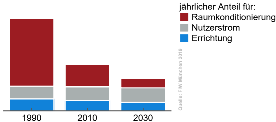
Abbildung 5: Qualitative Darstellung der Entwicklung des Primärenergiebedarfs eines typischen Gebäudes im Laufe der Zeit. Dargestellt sind die absoluten Anteile für Nutzerstrom, Raumwärme inklusive Warmwassererzeugung, sowie der Primärenergieeinsatz des Gebäudes für die Herstellungsphase der verwendeten Bauprodukte.
