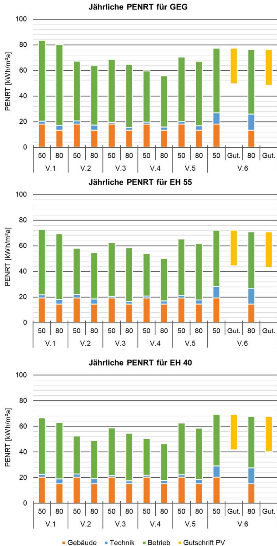
Abbildung 26: Jährliche PENRT für 50 und 80 Jahre Lebensdauer - GEG- EH55- EH40
