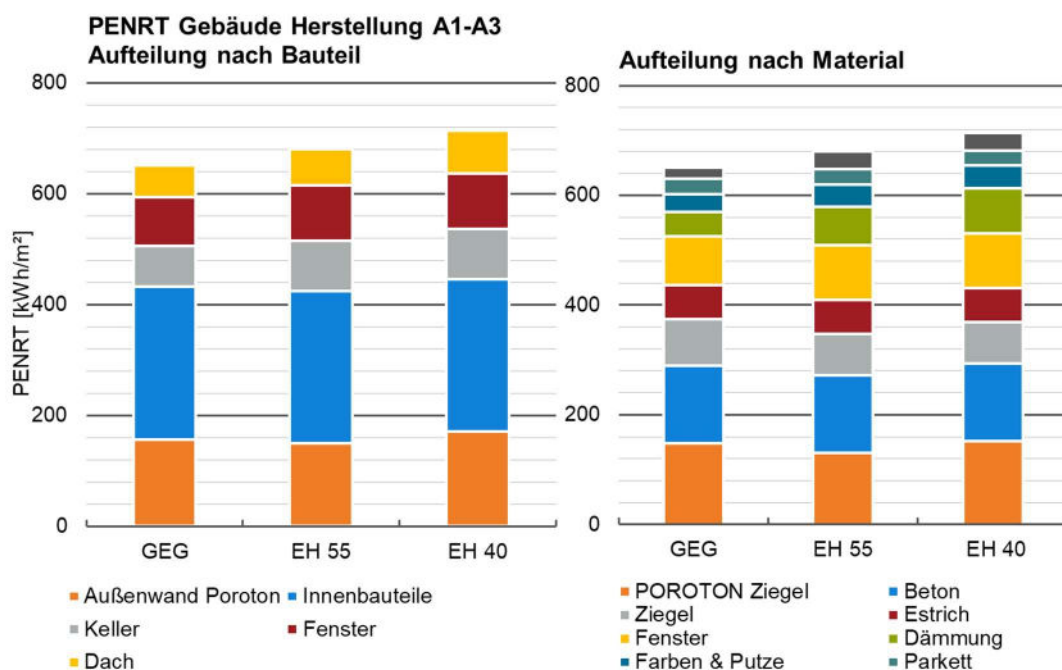
Abbildung 1: Vergleich der Grauen Energie nach Bauteilen und Material
