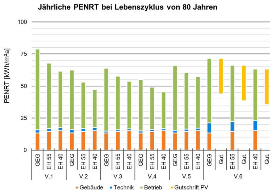
Abbildung 3: PENRT über den gesamten Lebenszyklus pro m² Nutzfläche für 80 Jahre Nutzungsdauer
