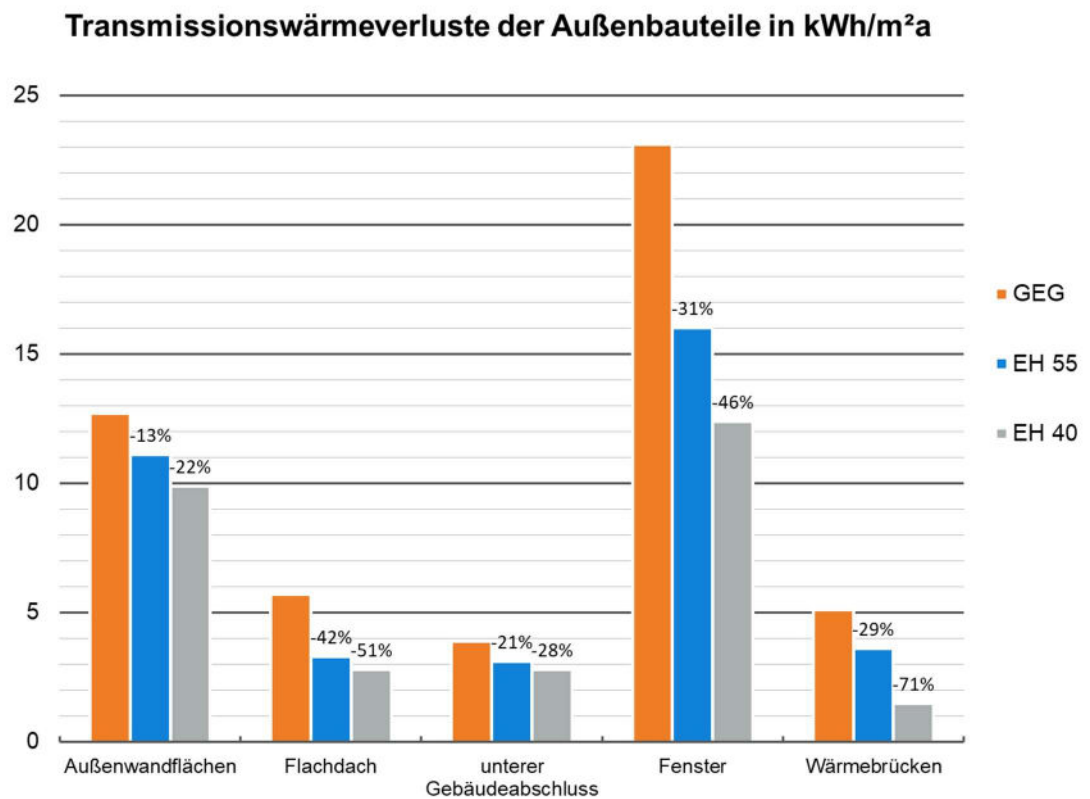
Abbildung 9: Transmissionswärmeverluste der Außenbauteile je Standard
