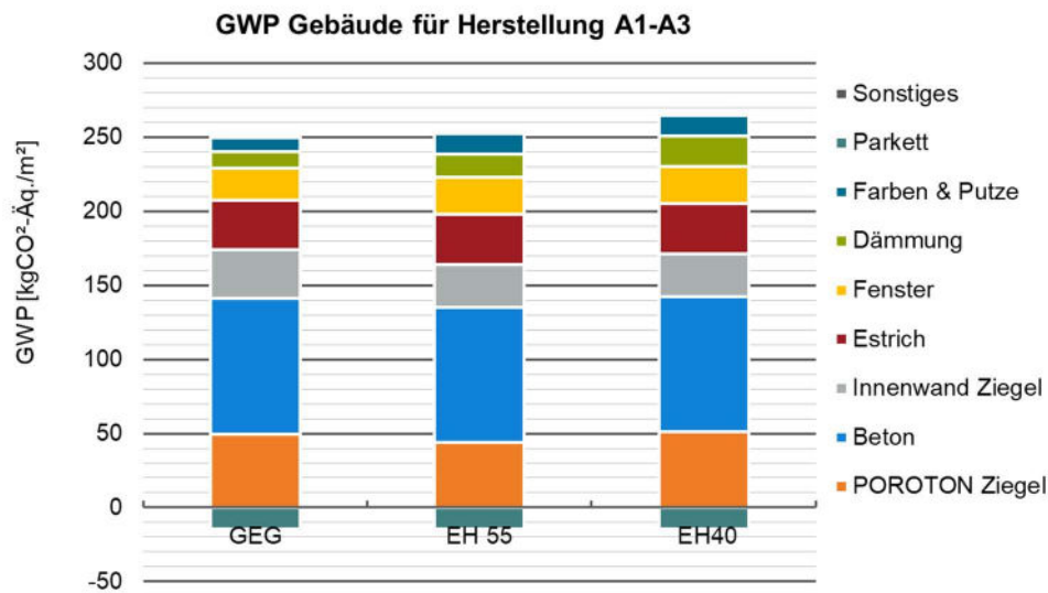
Abbildung 13: GWP Herstellungsphase A1-A3 für das Gebäude nach Material
