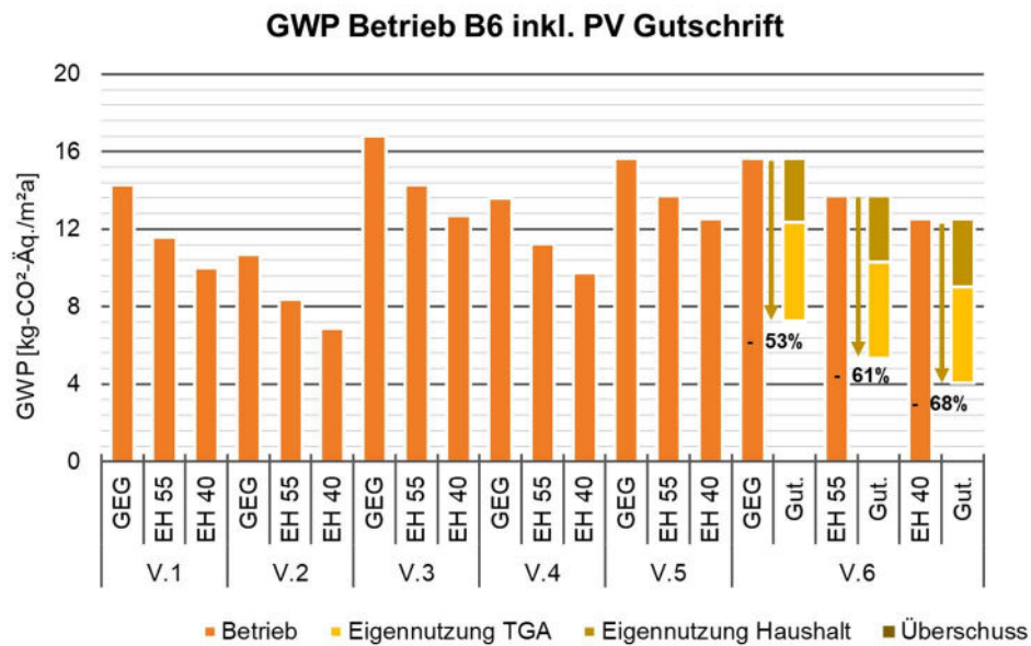
Abbildung 21: Jährliches GWP Betrieb B6 inkl. PV Gutschrift
