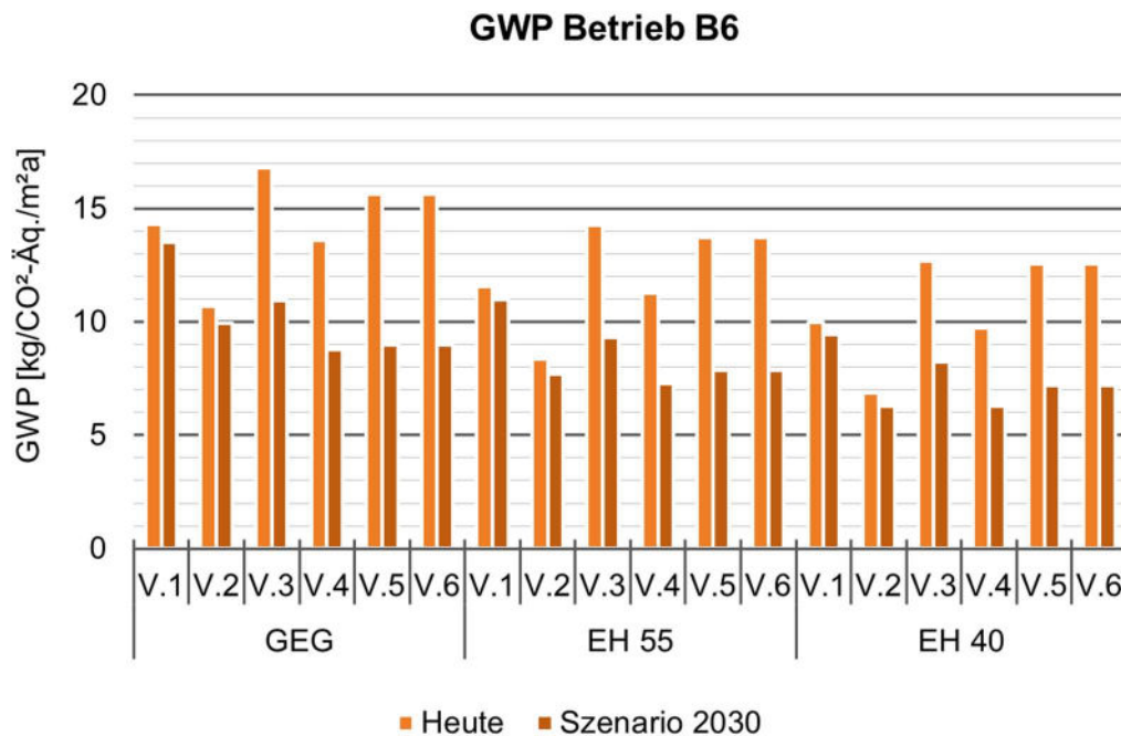
Abbildung 27: Jährliches GWP des Betriebs mit Faktoren für heute und 2030
