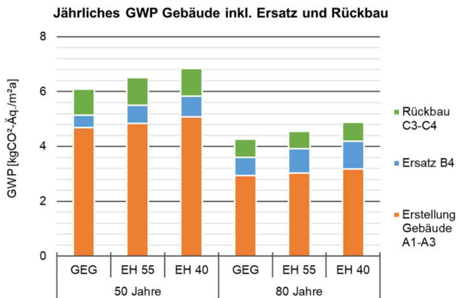
Abbildung 15: Jährliches GWP inkl. Ersatz und Rückbau für das Gebäude
