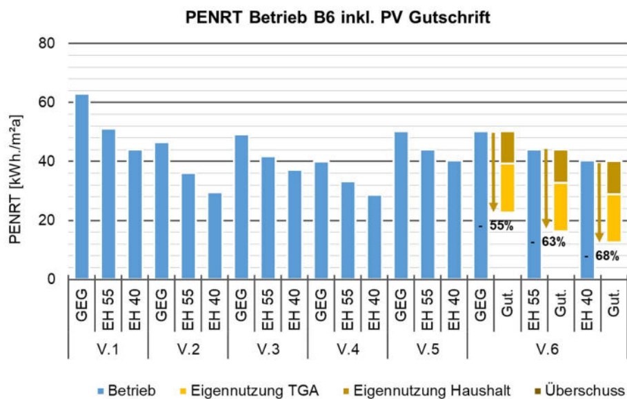
Abbildung 22: Jährliches PENRT Betrieb B6 inkl. PV Gutschrift
