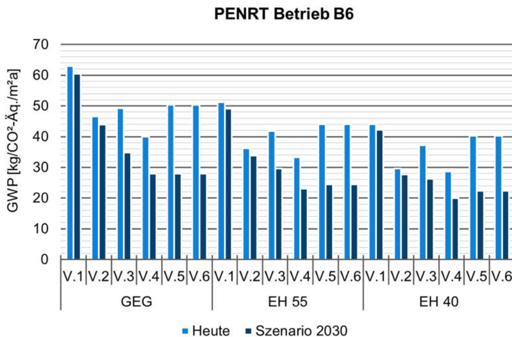
Abbildung 28: Jährliches PENRT im Betrieb für heute und 2030
