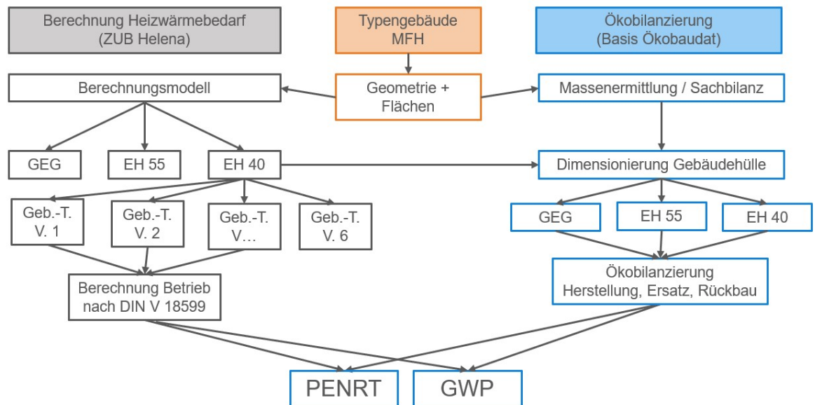
Abbildung 6: Schematisches Vorgehen im Rahmen der Studie
